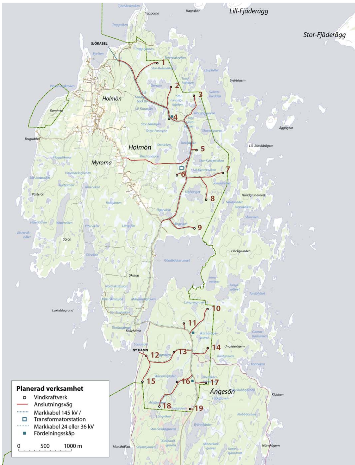
Figur 6. Planerad utformning av verksamheten med vindkraftverk 1-19, vägar (röda linjer) och ny hamn vid verk 12. Kraftledningarna kommer att läggas i mark längs vägnätet. De exakta placeringarna av vindkraftverk och vägar kan komma att ändras till tillståndsansökan.
